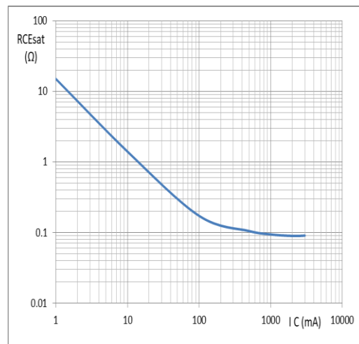
R CE(sat) - I C
