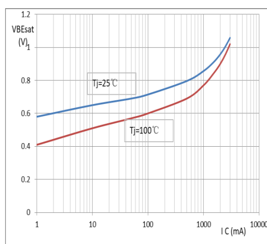
V BE(sat) - I C
